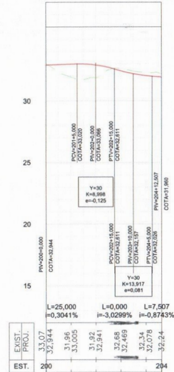
PERFIL LONGITUDINAL - R-200
