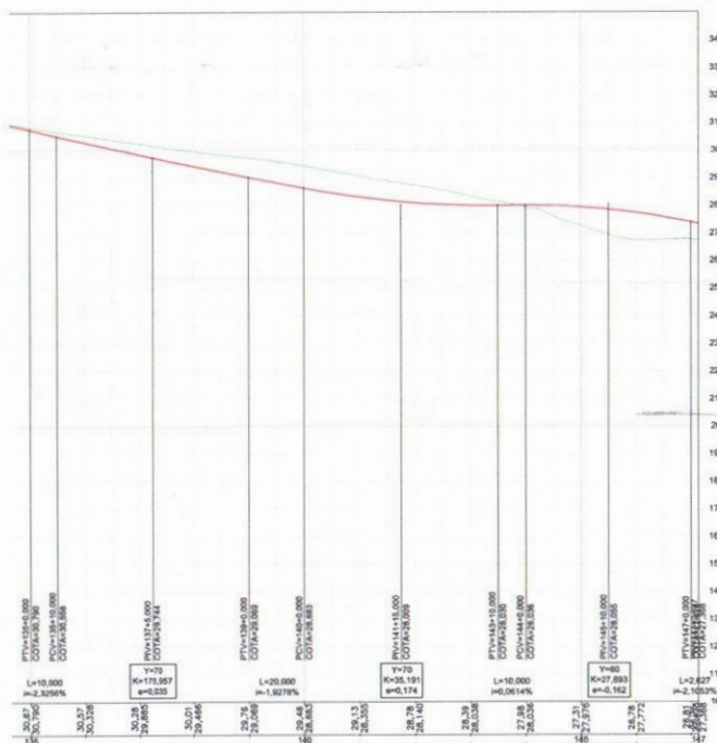
PERFIL LONGITUDINAL - SEN_R-300
