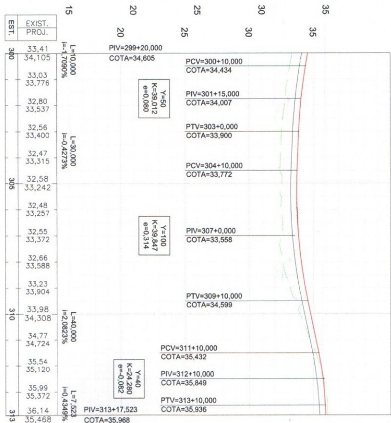
PERFIL LONGITUDINAL- R-300
