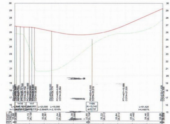
PERFIL LONGITUDINAL - SES_R-400
