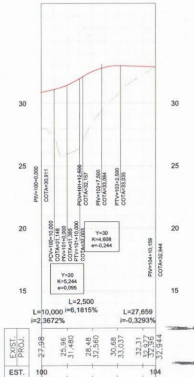
PERFIL LONGITUDINAL - R-100
