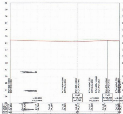
PERFIL LONGITUDINAL - SES_R-300
