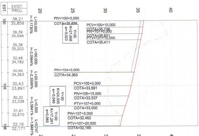
PERFIL LONGITUDINAL- R-100
