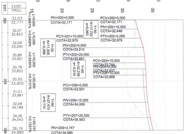
PERFIL LONGITUDINAL- R-200
