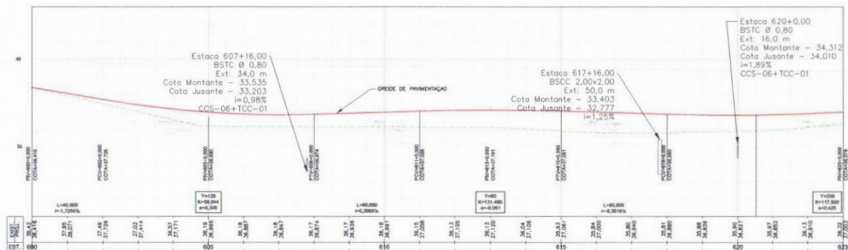
PERFIL LONGITUDINAL - EIXO-BR-101
