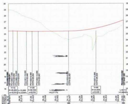
PERFIL LONGITUDINAL - SEN_R-300
