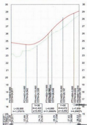
PERFIL LONGITUDINAL - SEN_R-400
