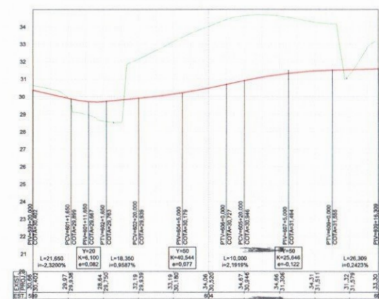
PERFIL LONGITUDINAL - SEN_R-600
