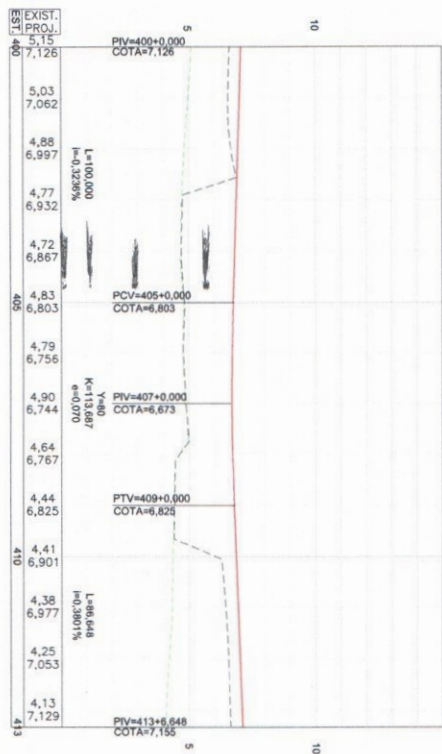
PERFIL LONGITUDINAL - RAMO-400
