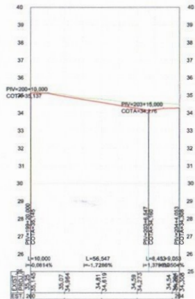
PERFIL LONGITUDINAL - SES_R-200
